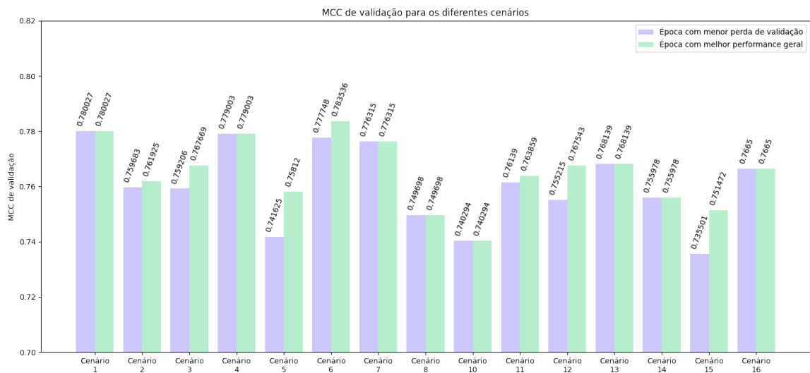
Figura 5.9: Valores do coeficiente de correlação de Matthews de validação para os cenários selecionados.
