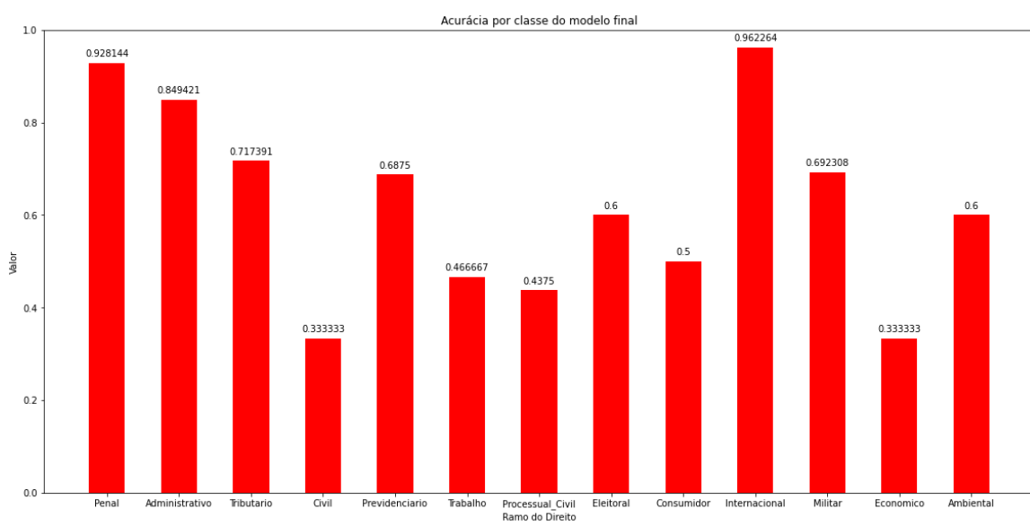
Figura 5.13: Valores de acurácia por ramo do Direito para o modelo do cenário 1 no conjunto de dados de teste.
