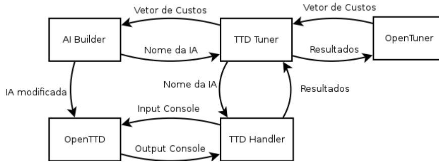
Figura 4.1: Estrutura do tuner implementado
