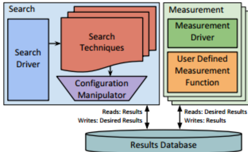
Figura 2.1: Diagrama de Funcionamento do OpenTuner
